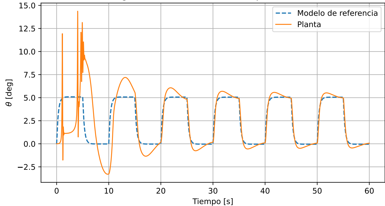
Seguimiento MRAC con tren de pulsos: theta
